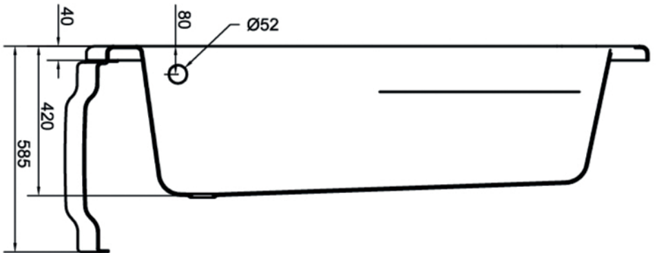
A-A (1 : 10)
